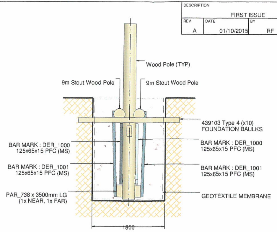
LONGITUDINAL ELEVATION
